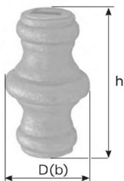
E4/009A-14,5x14,5 h67, D45
